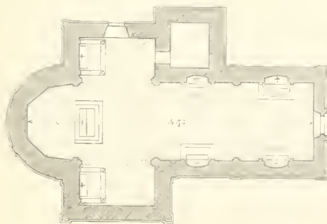
Kirche zu Castel Nigone
